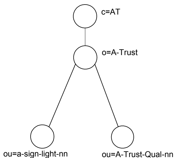
Abbildung 2 a.trust Verzeichnisbaum
